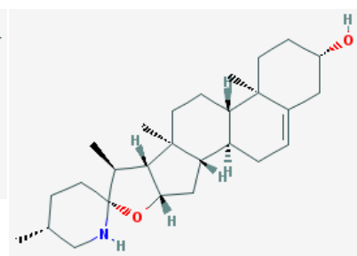
Solasodine
