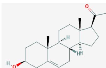
Pregnenolone
