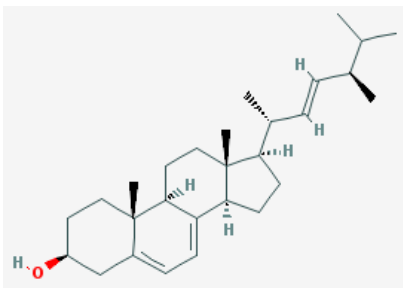
Ergosterol
