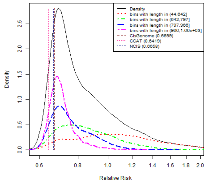
(d) CTCF, K = 2000
