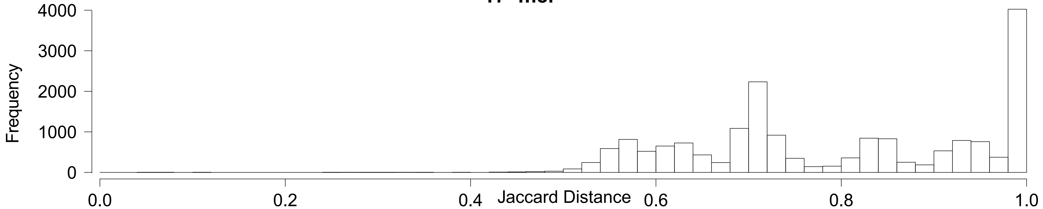
21-mer
