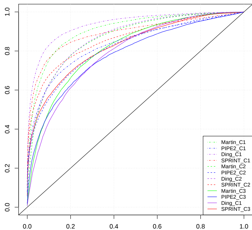
MINT (C123, ROC)
