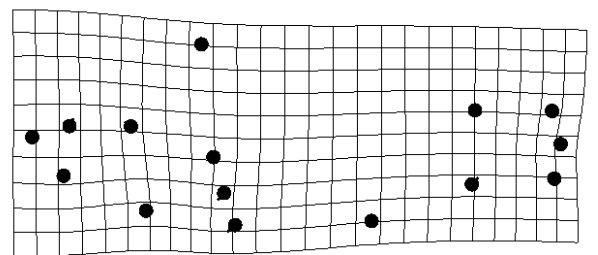
anc -- maf
