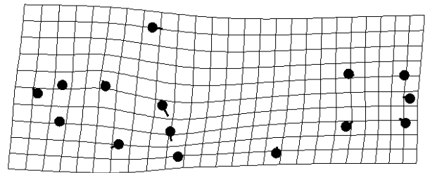
anc -- kig
