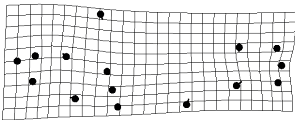
anc -- kaw
