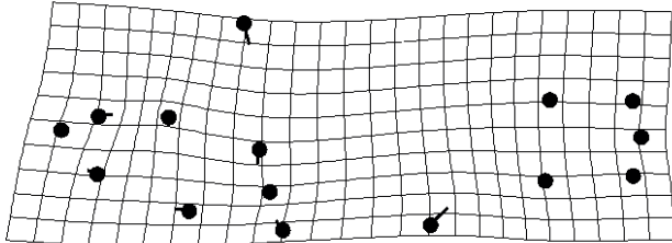
anc -- kat
