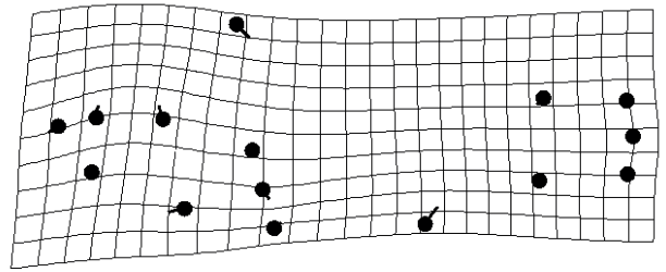
anc -- chi
