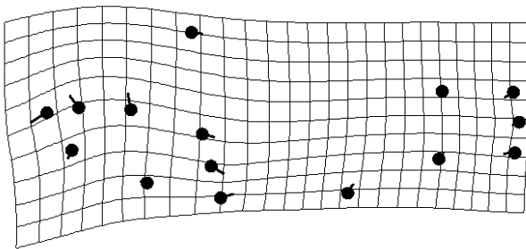
anc -- nku
