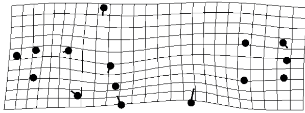
anc -- kab
