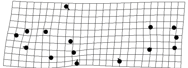
anc -- mug
