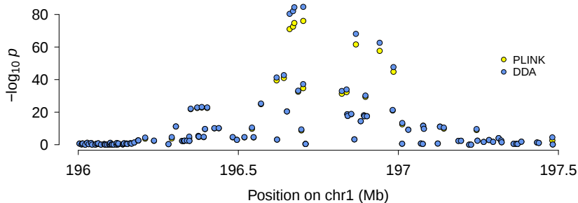
B: C2/CFB
