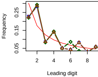
50bp(SE)
