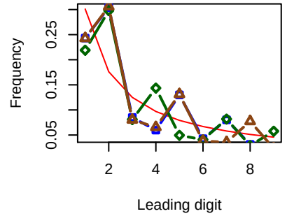
25bp(SE)
