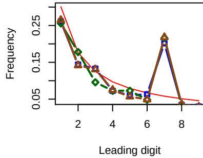
30%(SE)
