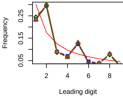
80%(SE)
