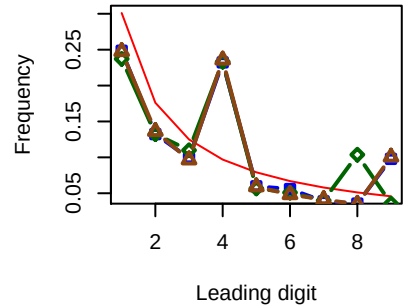
50%(SE)
