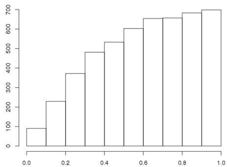
MIA3 #1
