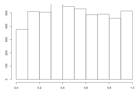
MRAS
