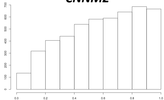
CNNM2
