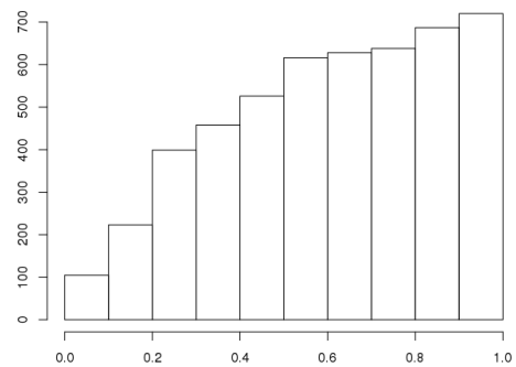
MIA3 #2
