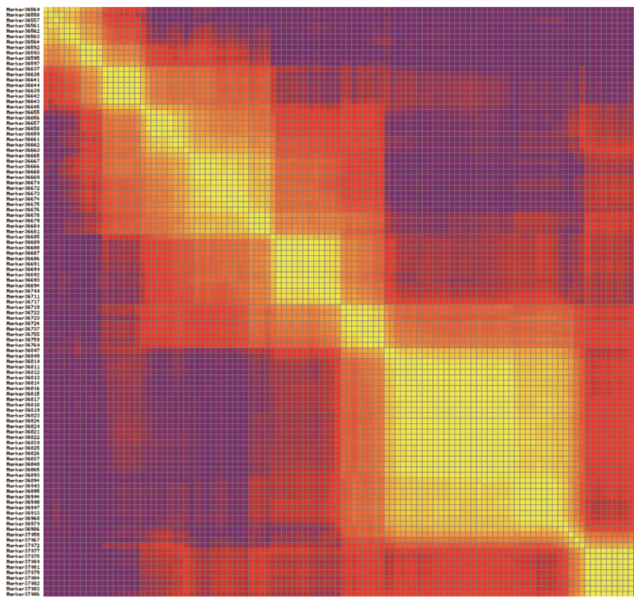
Chromosome D11
