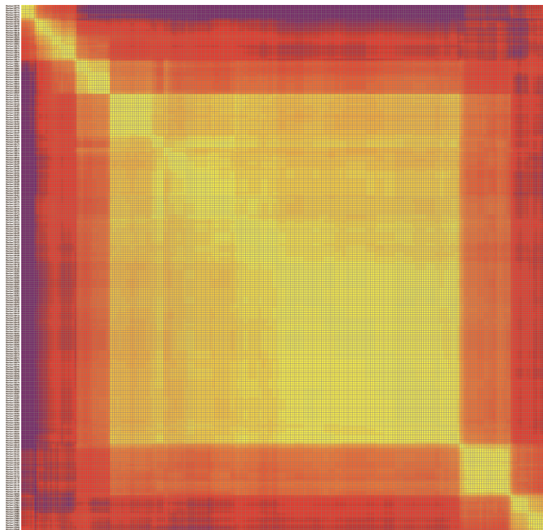
Chromosome D13
