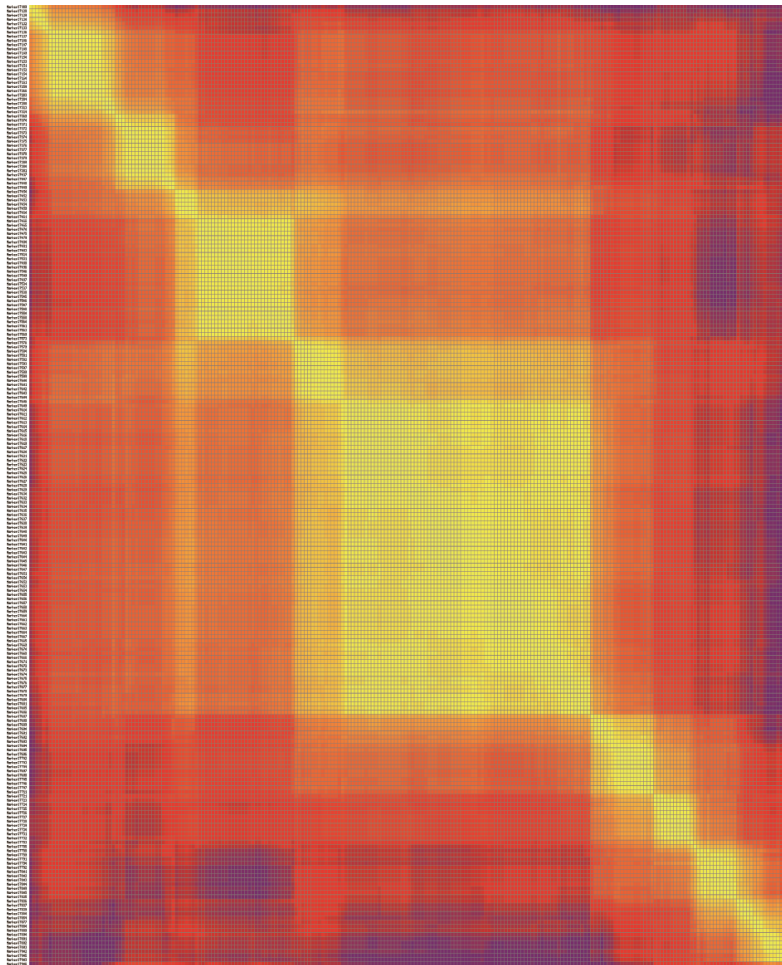
Chromosome D12
