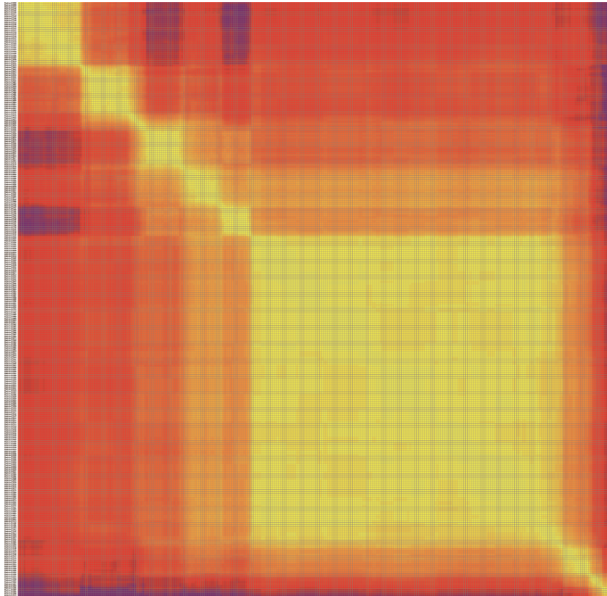
Chromosome A7
