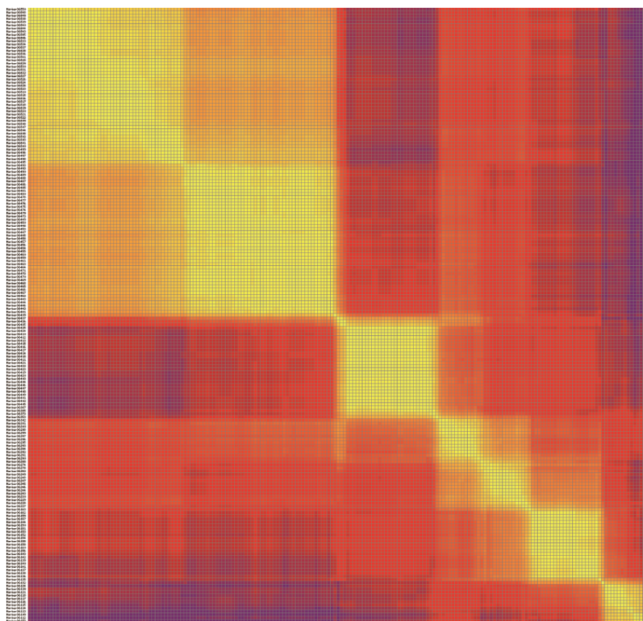
Chromosome D10
