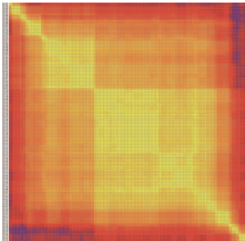
Chromosome D2
