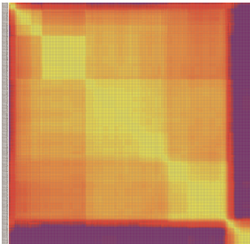
Chromosome D1
