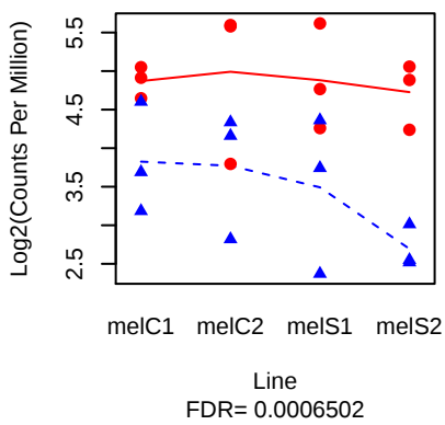
TotZ ( FBgn0044809 )
