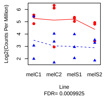
et ( FBgn0031055 )
