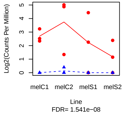
Hsc70-1 ( FBgn0001216 )
