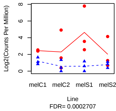
Drs ( FBgn0010381 )
