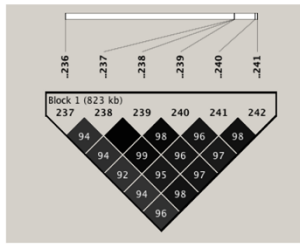
18:1 Chr6
