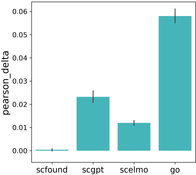
CollecTRI
