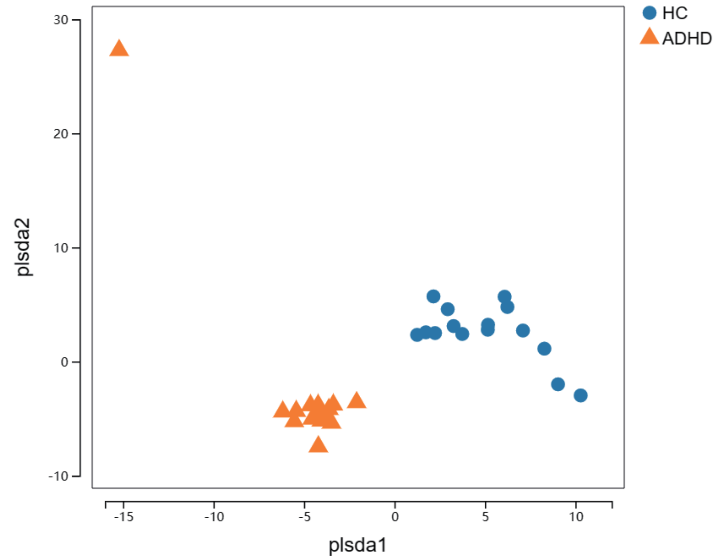
PLS-DA
