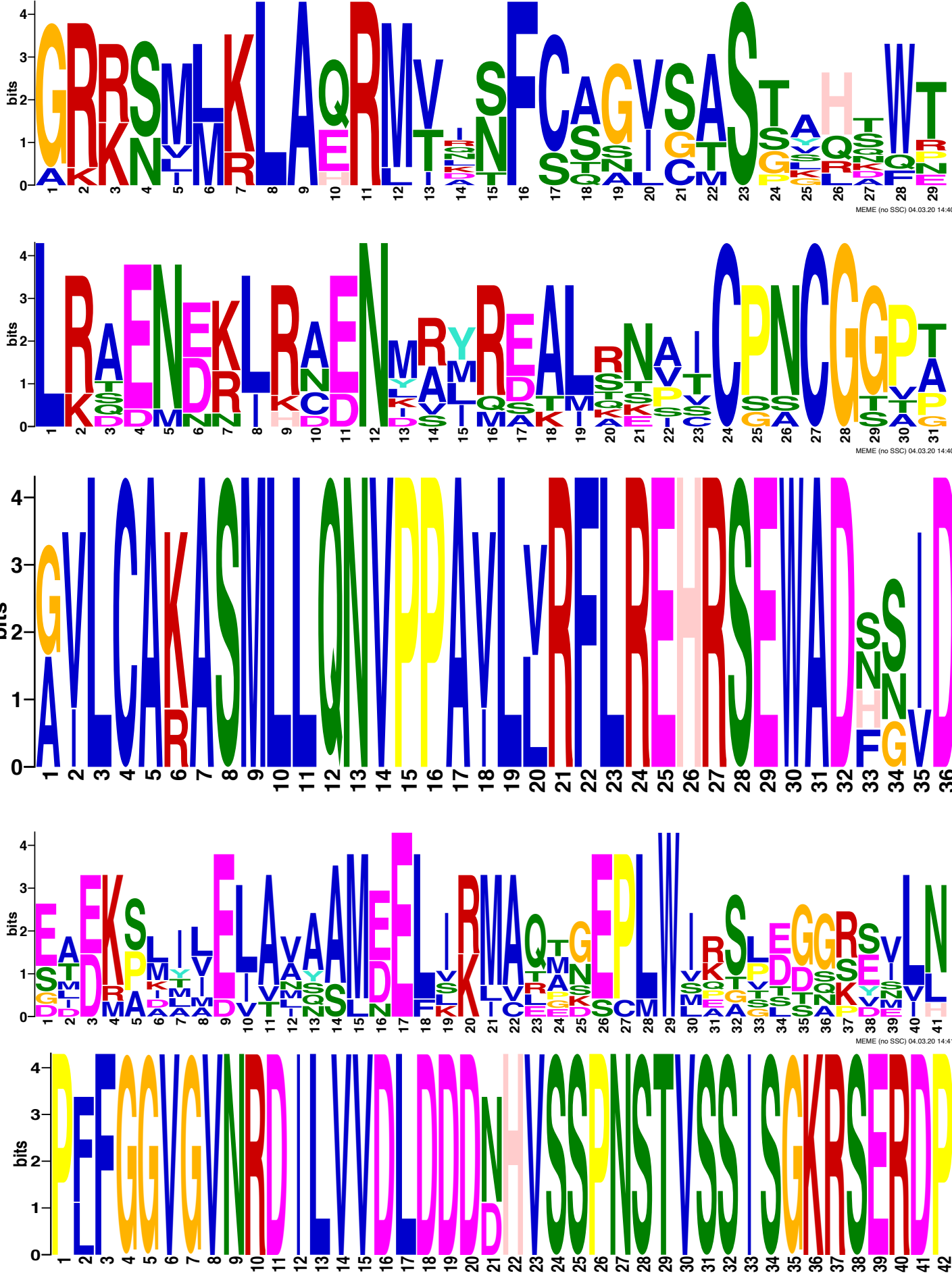
Motif 16
