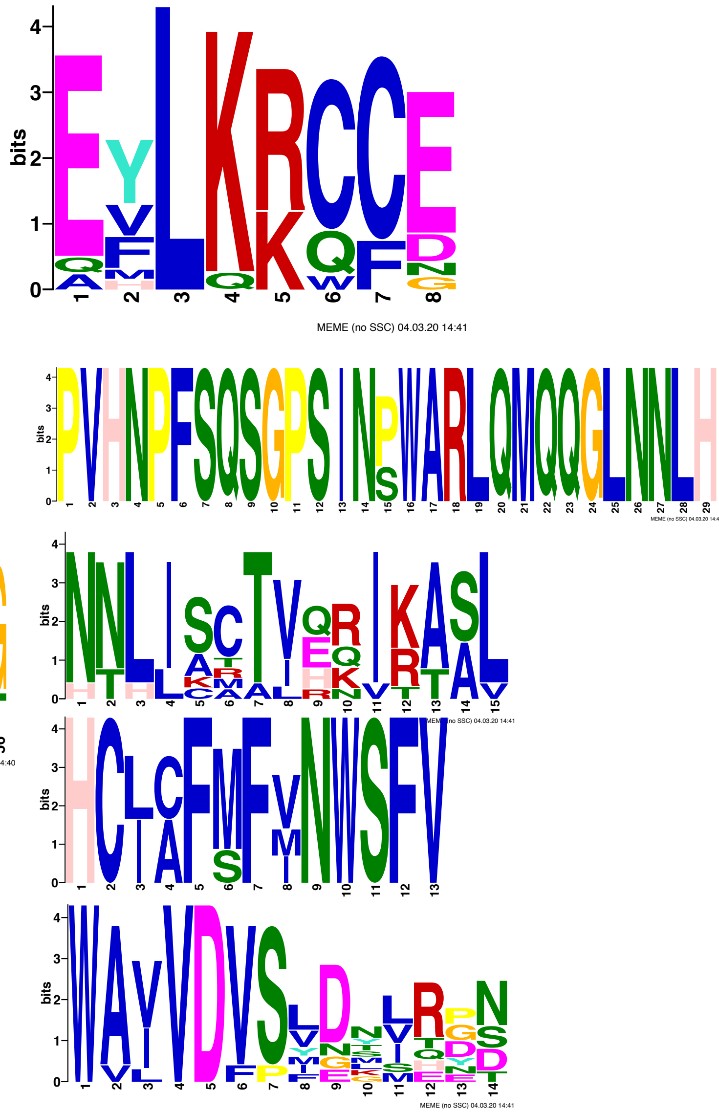
Motif 21
