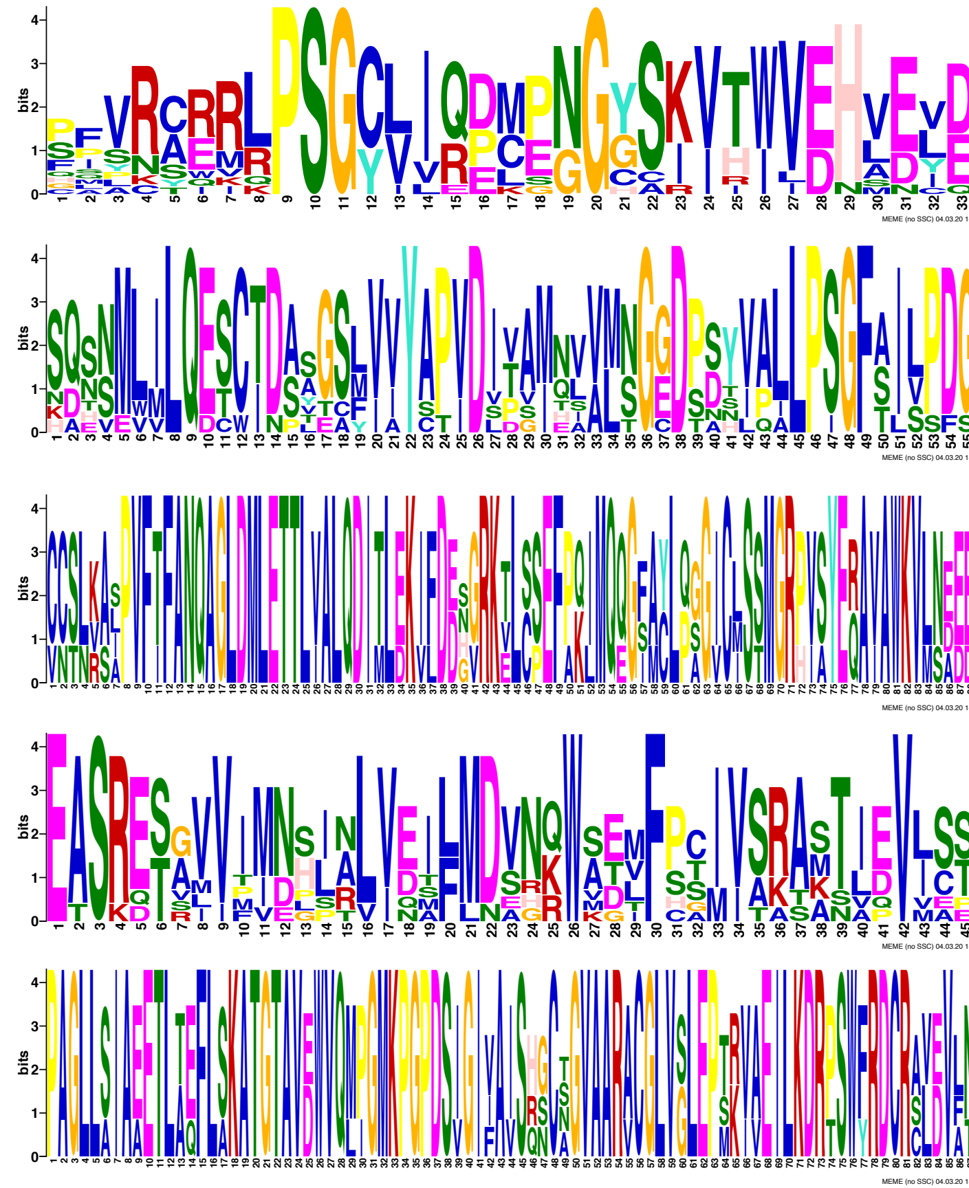
Motif 6
