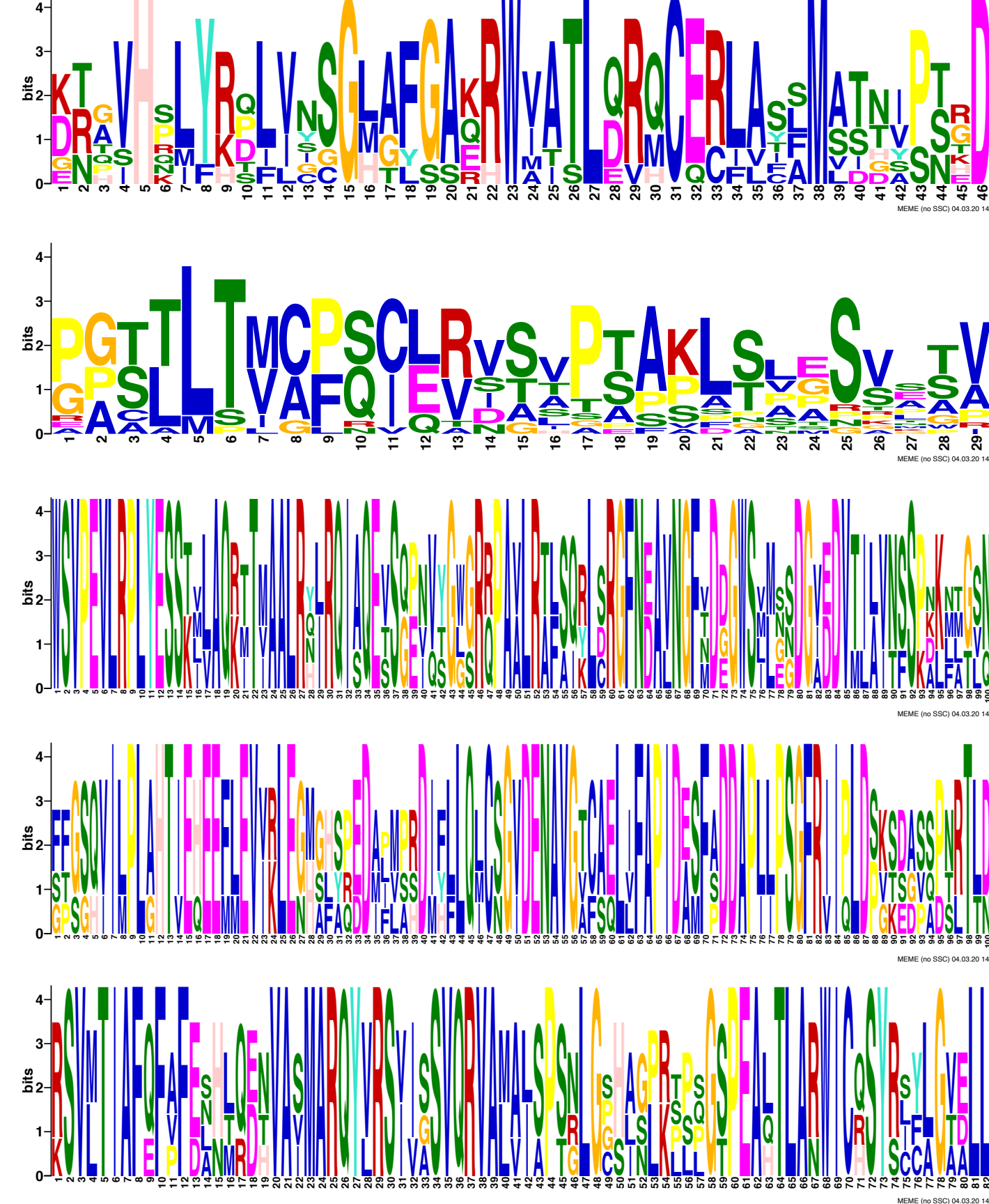
Motif 11
