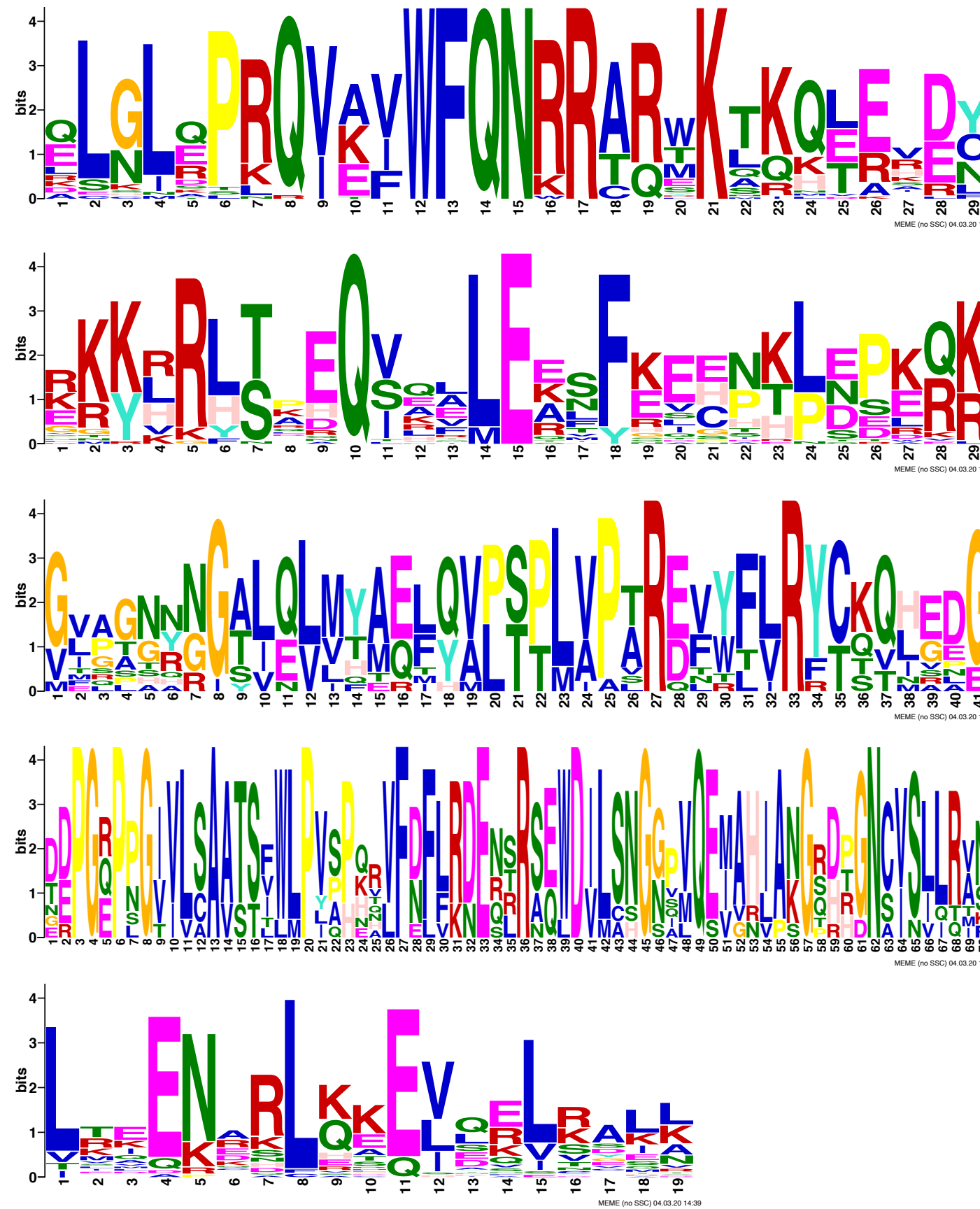
Motif 1
