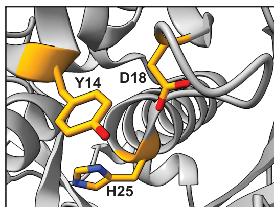
EcYbgC (PDB ID 5T06)
