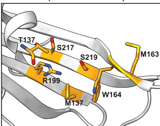
UcFatB N-term. (PDB ID 5X04)
