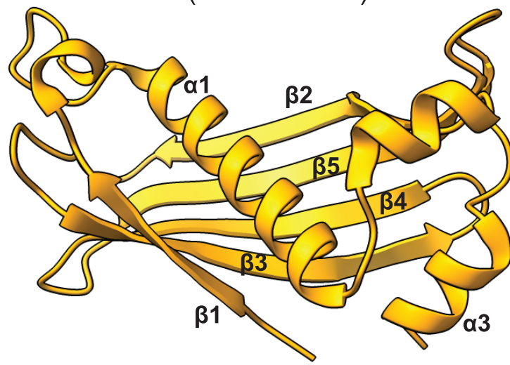
EcYbgC (PDB ID 5T06)
