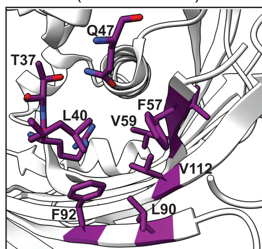
EcYbgC (PDB ID 5T06)
