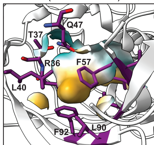
UcFatB N-term. (PDB ID 5X04)
