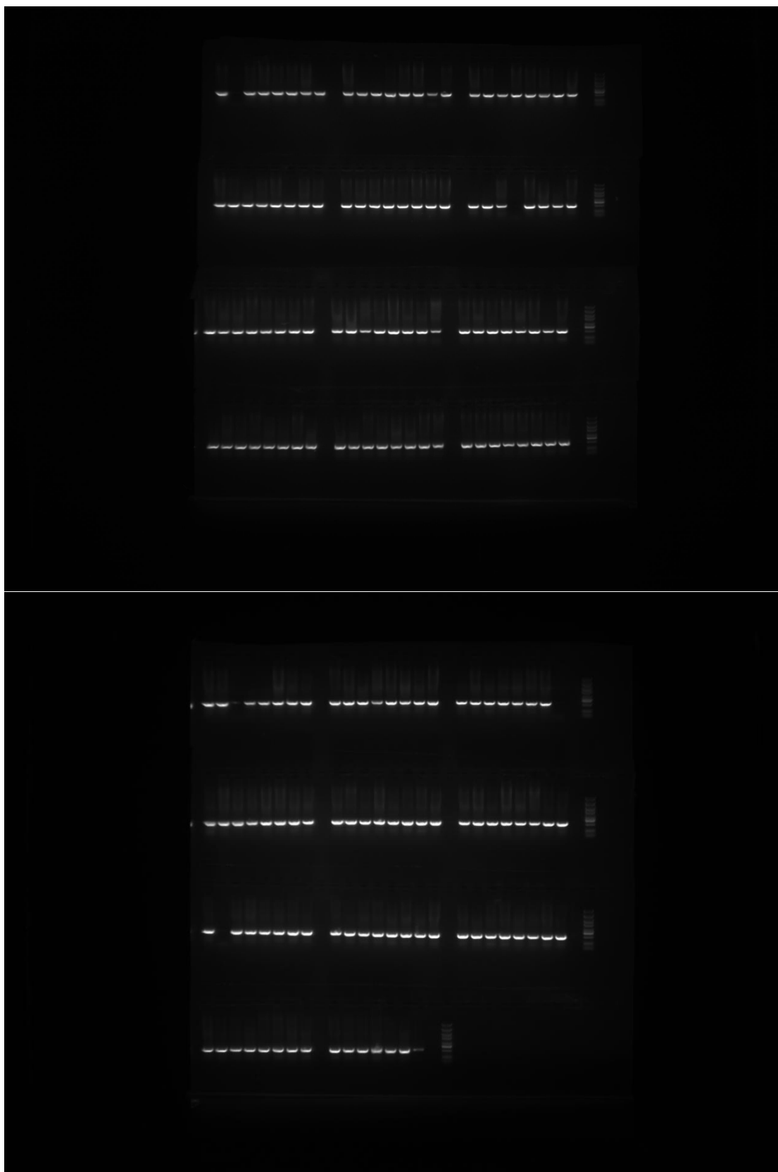
trnL-trn F
