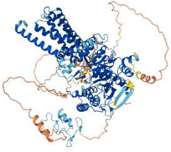
BnCesA1
