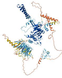
BnCesA5
