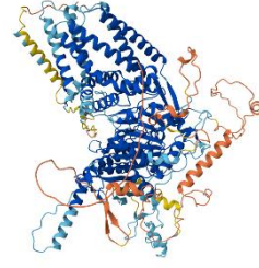
BnCslD1
