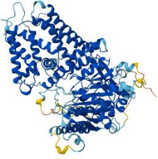
BnCslB2
