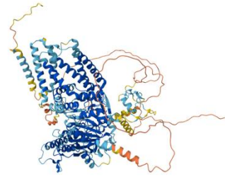
AtCesA4
