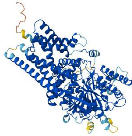
BnCslG1
