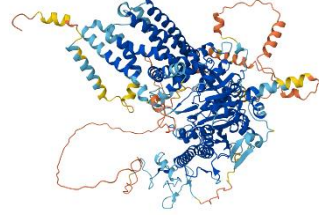
BnCslA3
