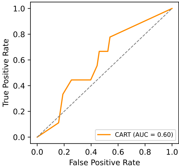
CART ROC (test set, n=72)
