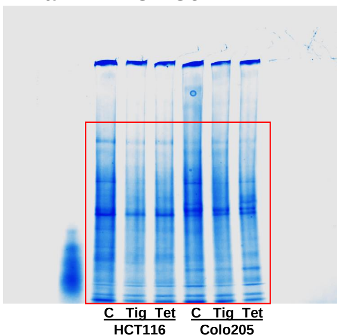
B. a. BN-PAGE Gel
