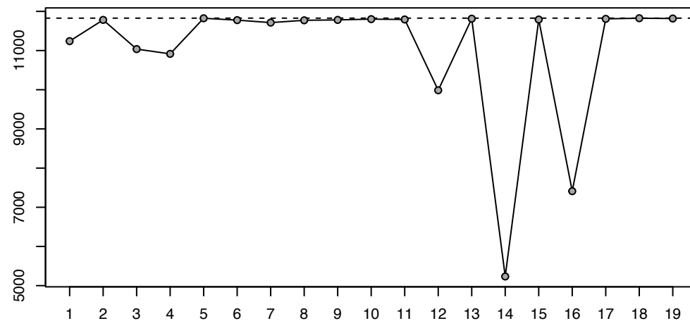
QE.del
