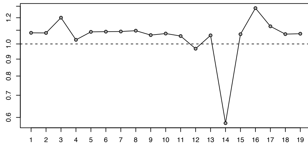
cov.r
