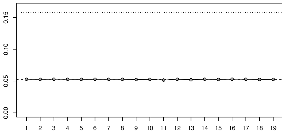
hat
