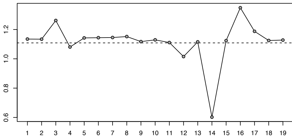
tau2.del
