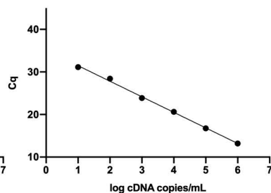
Actb
