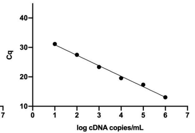
Rpl13a
