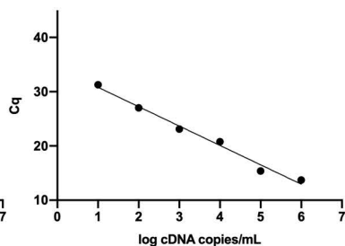
Rpl13a
