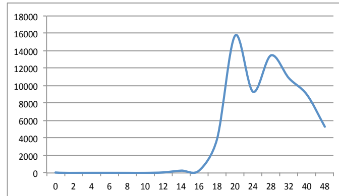
NvfoxD3 Cp_0hpf: 40.00
