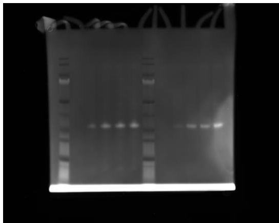
G. 0.0125 mM IPTG flask #3
