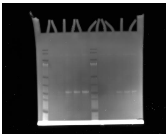
E. 0.1 mM IPTG flask #5 – AaSPI-NL
