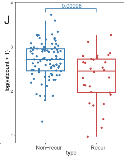
HECTD4
