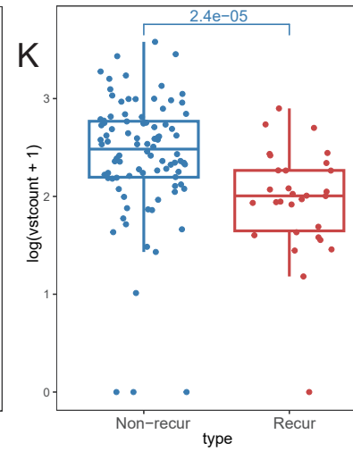
ACTRT2
