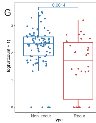
ACTRT2
