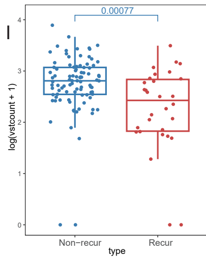
LLPH
