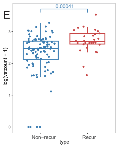
LLPH
