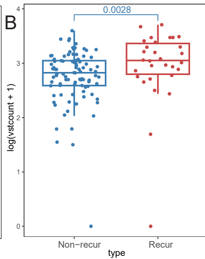
ANGPT2
