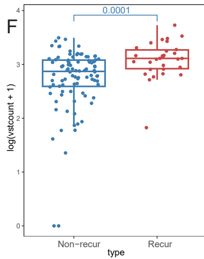
HECTD4
