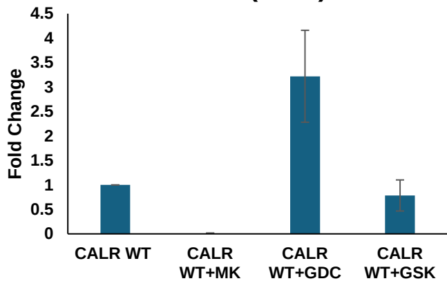
AKT (S473)
