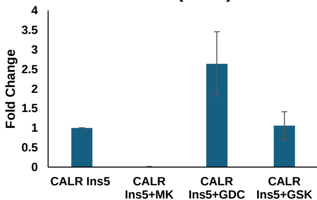
AKT (S473)
