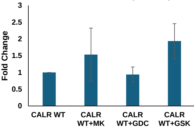
mTORC1(S2448)
