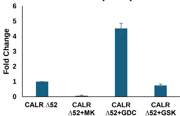
AKT (S473)
