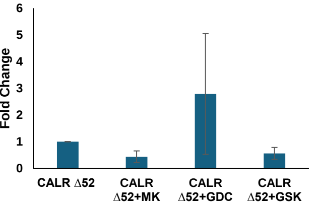
mTORC1(S2448)
