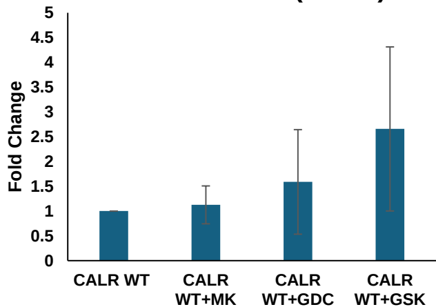
mTORC2(S2481)
