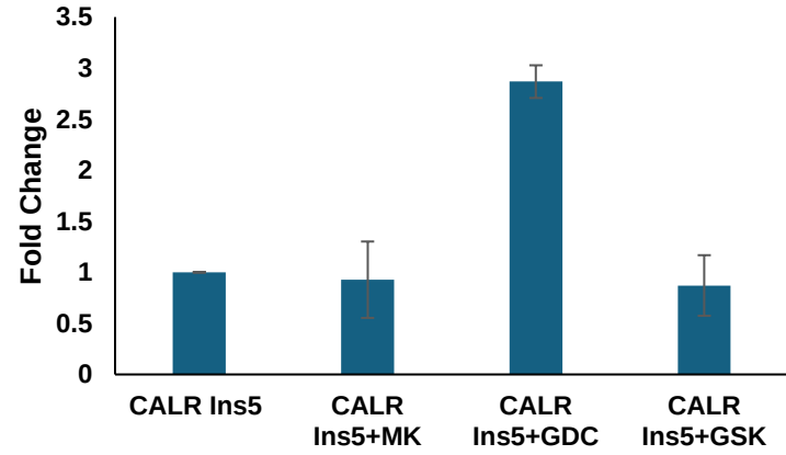
AKT (T308)
