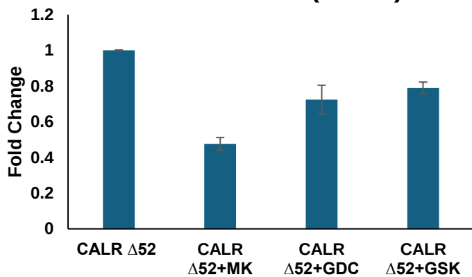
mTORC2(S2481)
