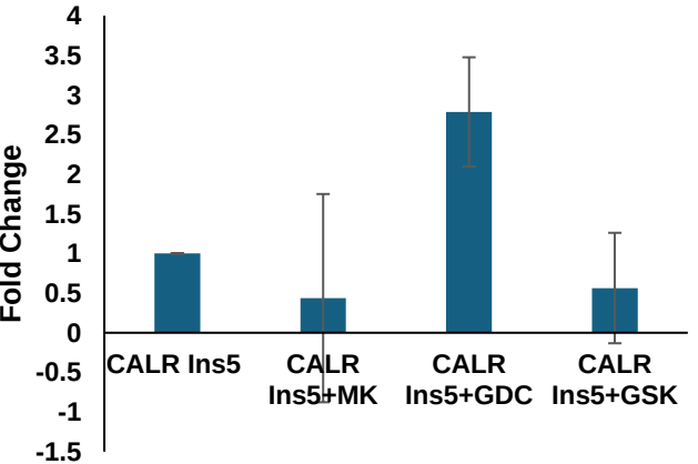
mTORC1(S2448)
