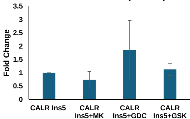
mTORC2(S2481)
