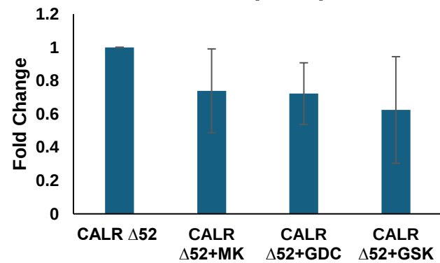
AKT (T308)
