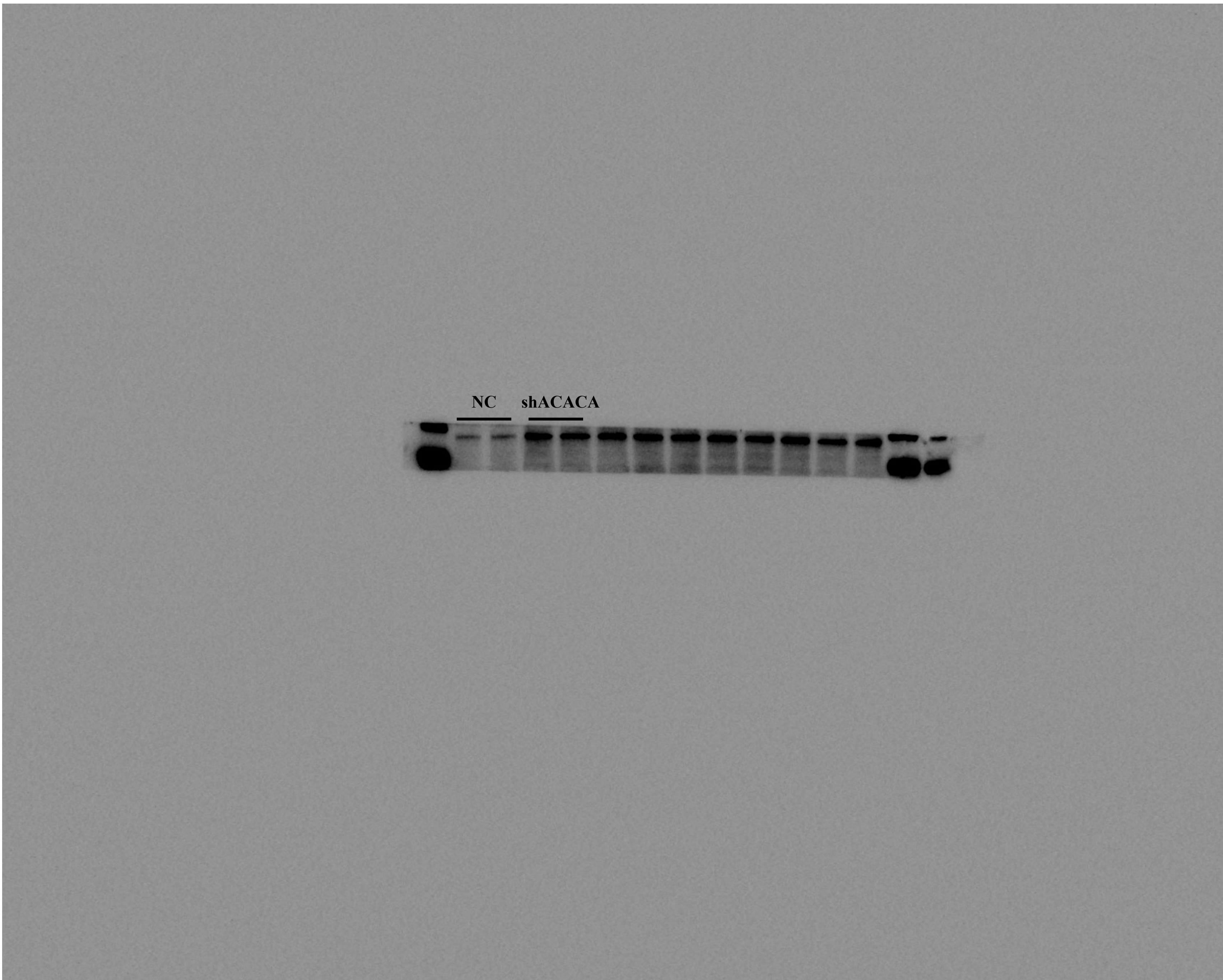
Figure 7A IKKα
