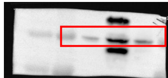
TGF-β 1 33KDa
