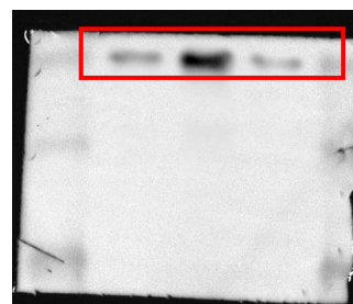
p-p38 43KDa
