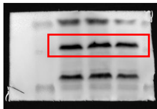
p38 43KDa
