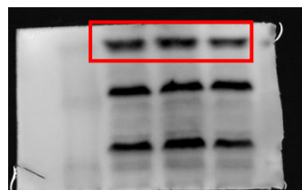
p38 43KDa
