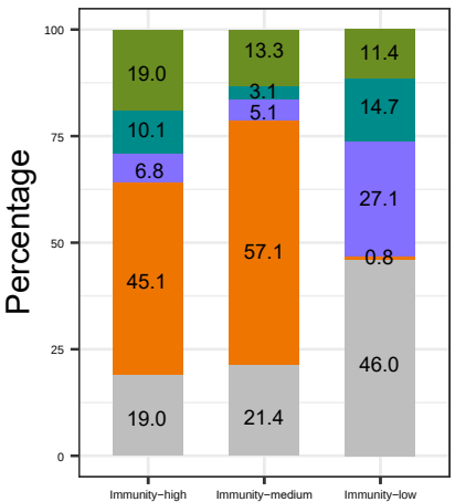
TCGA-glioma
