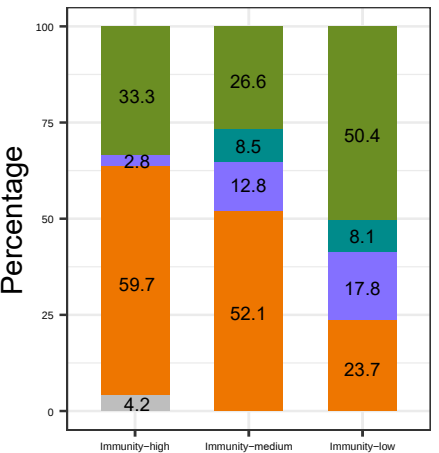
CGGA301
