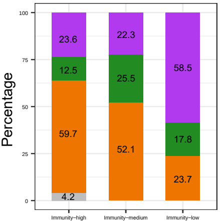
CGGA301
