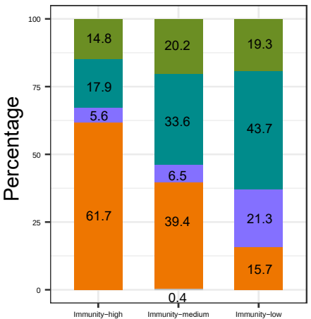
CGGA693
