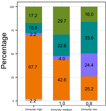
CGGA325
