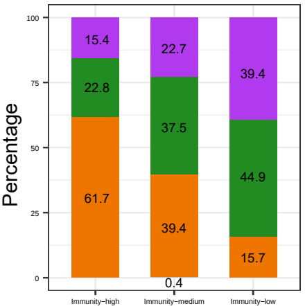
CGGA693
