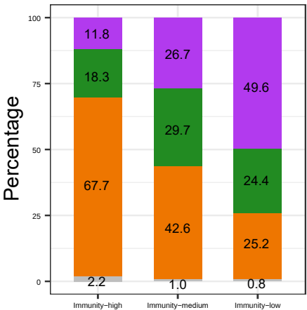
CGGA325
