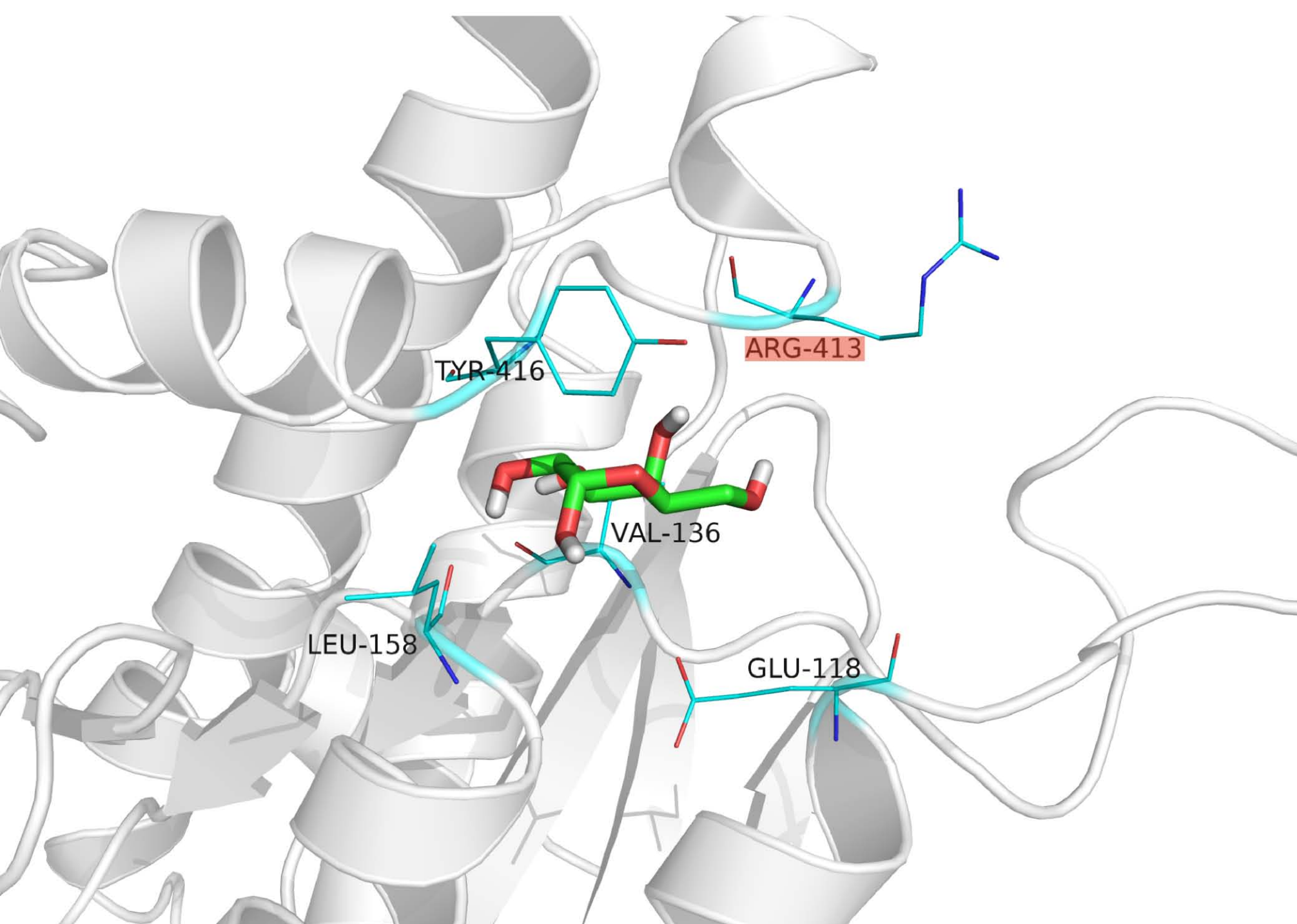
D-galactose
