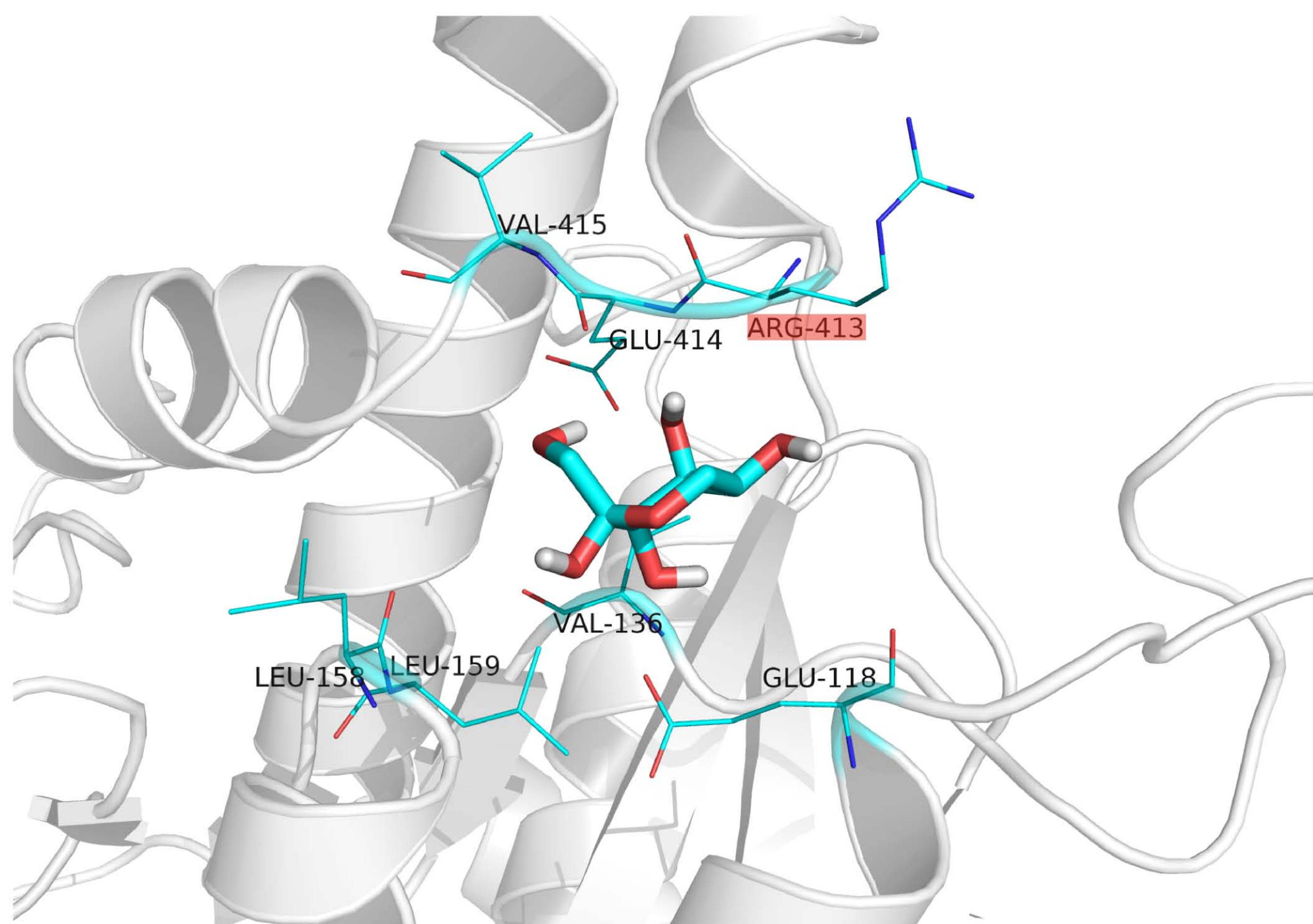
fructose
