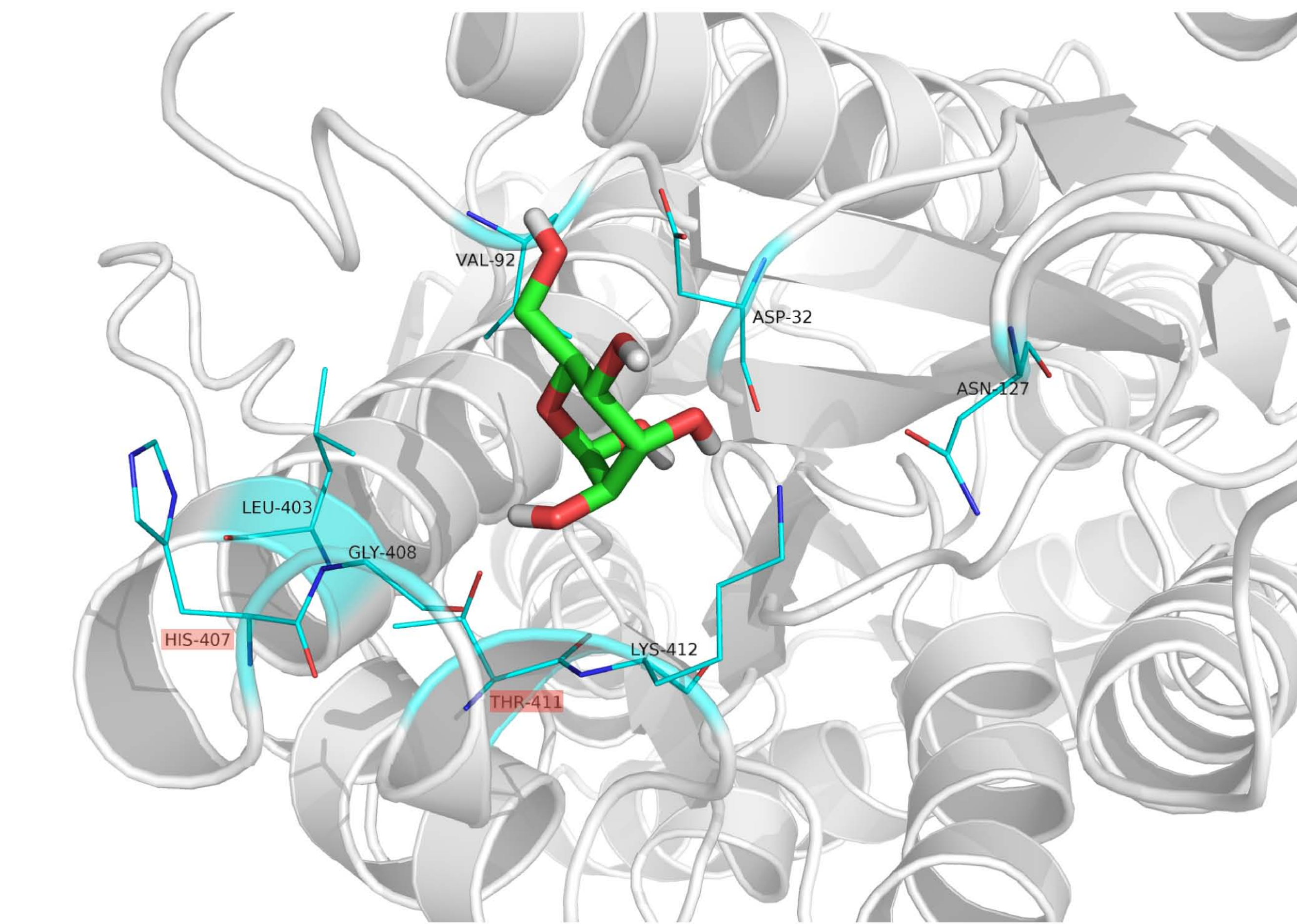
galactose
