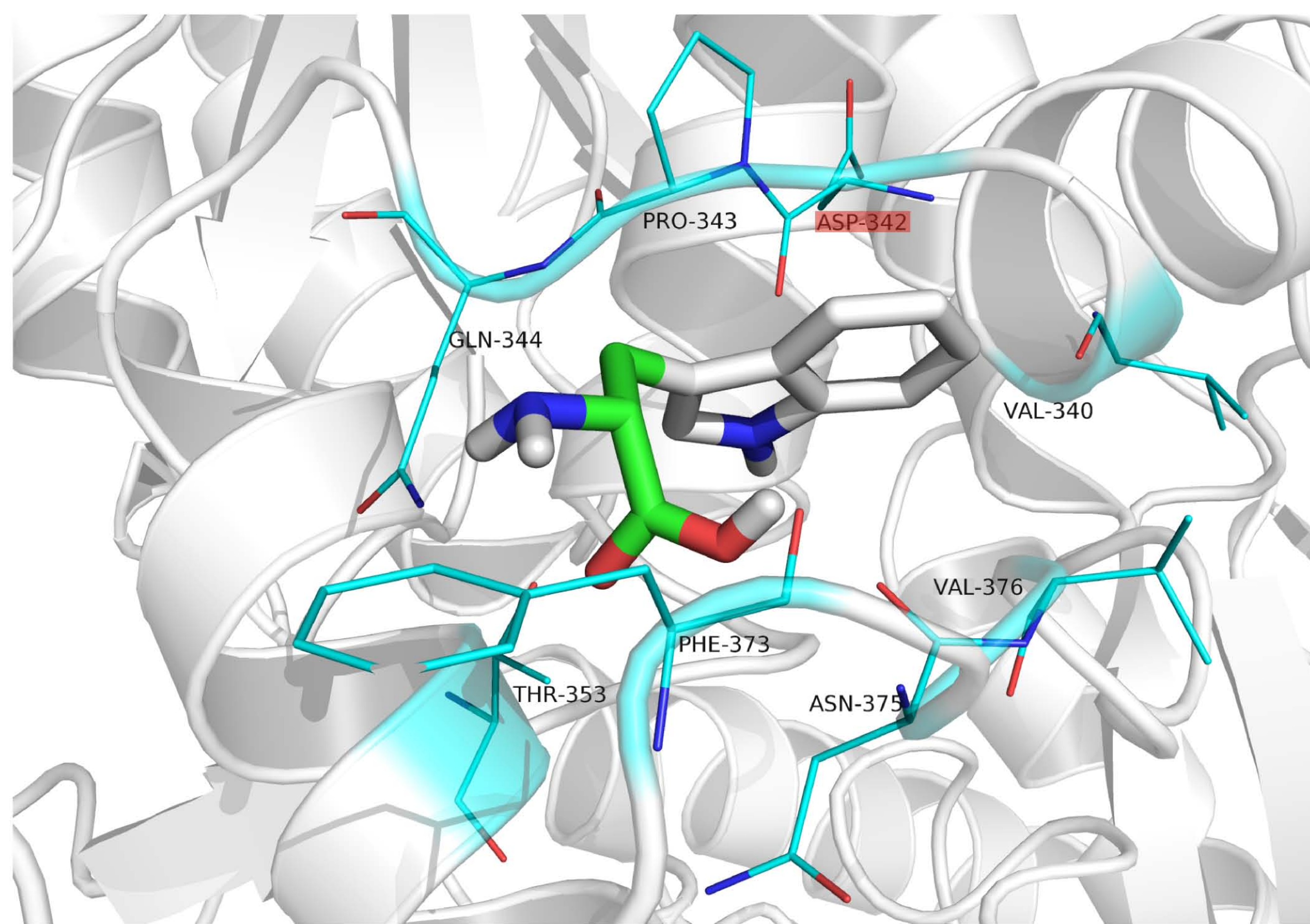
D-tryptophan
