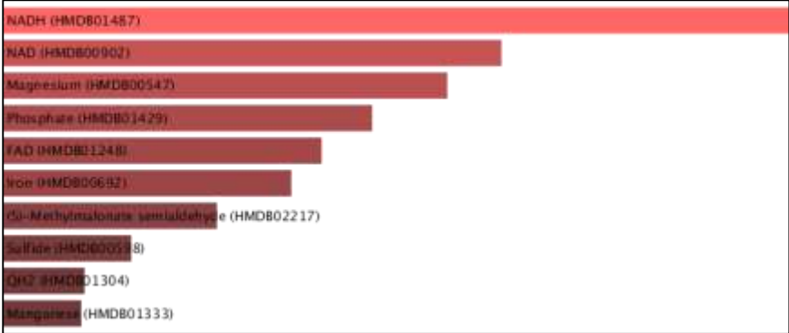
f. HMDB
