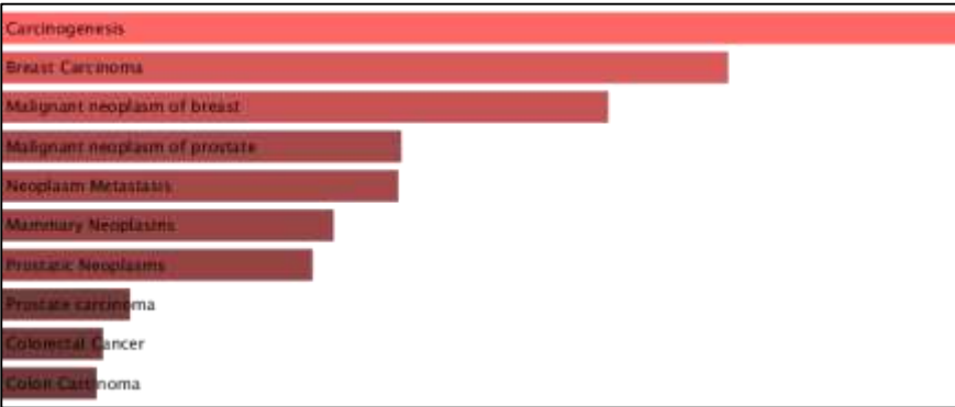
e. DisGeNET
