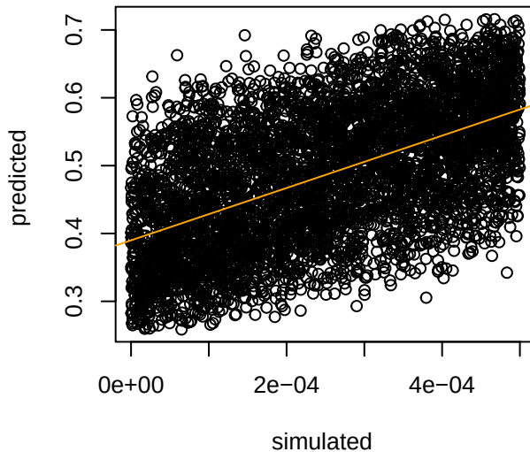
migrationNAfb_WAf
