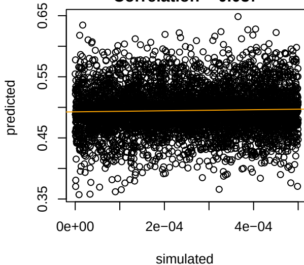
migrationEU_ME
