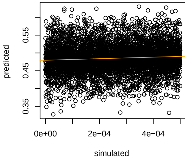
migrationNAfb_to_ME
