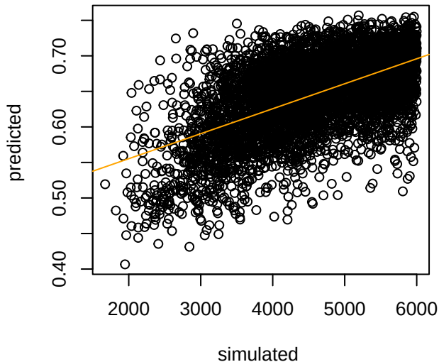
tNAfb_NAfa_ME_EU_BEi_EAs_WAf
