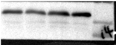
Sirt1
