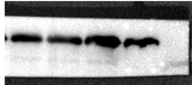
Sirt1
