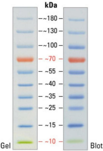
4-20% Tris-glycine SDS-PAGE
