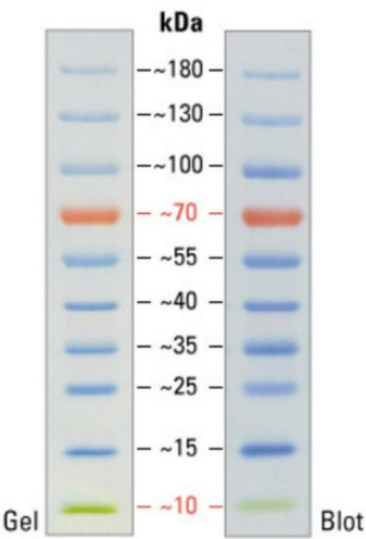
4-20% Tris-glycine SDS-PAGE
