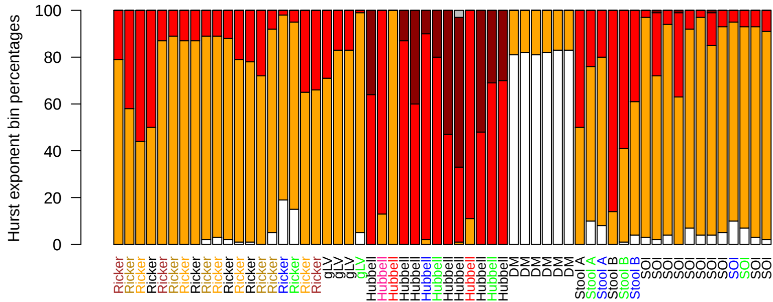
b) Hurst exponent
