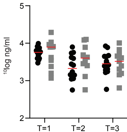
Unbound IgA
