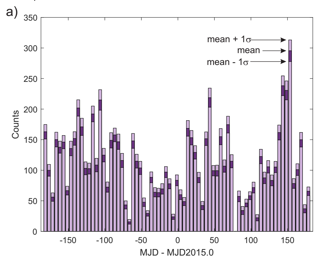
IGRF parent model
