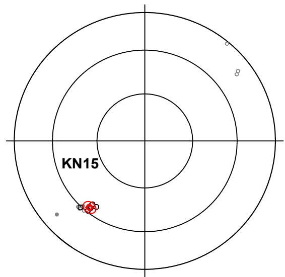
Königsberg (Tieschen)
