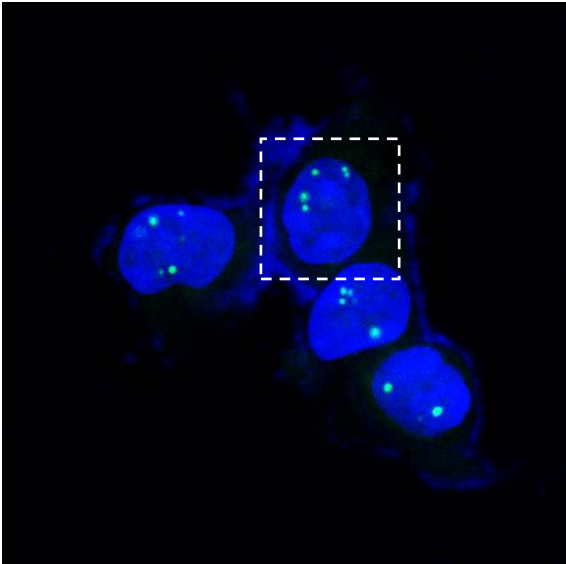
siARID1B
