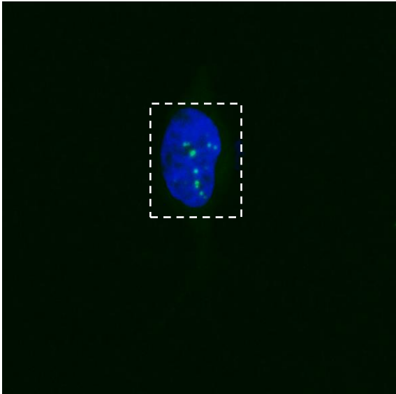
siScramble
