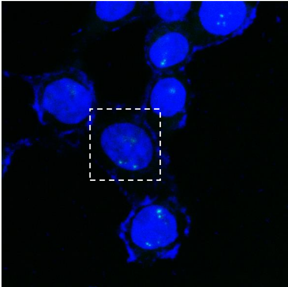
siNONO
