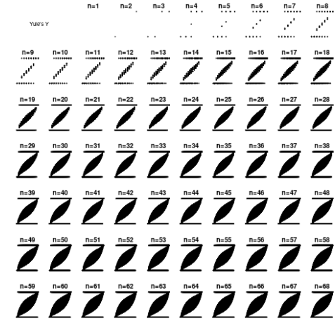
Fig. 13 Yule's Y
