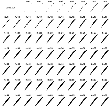
Fig. 6 Gwet's AC1
